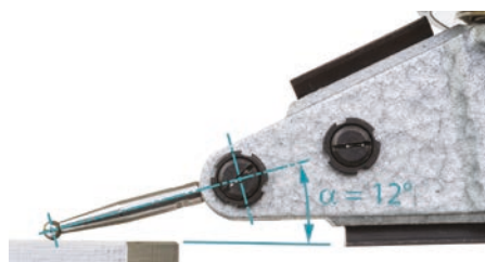
Hrot doteku s úhlovou pozicí 12°
